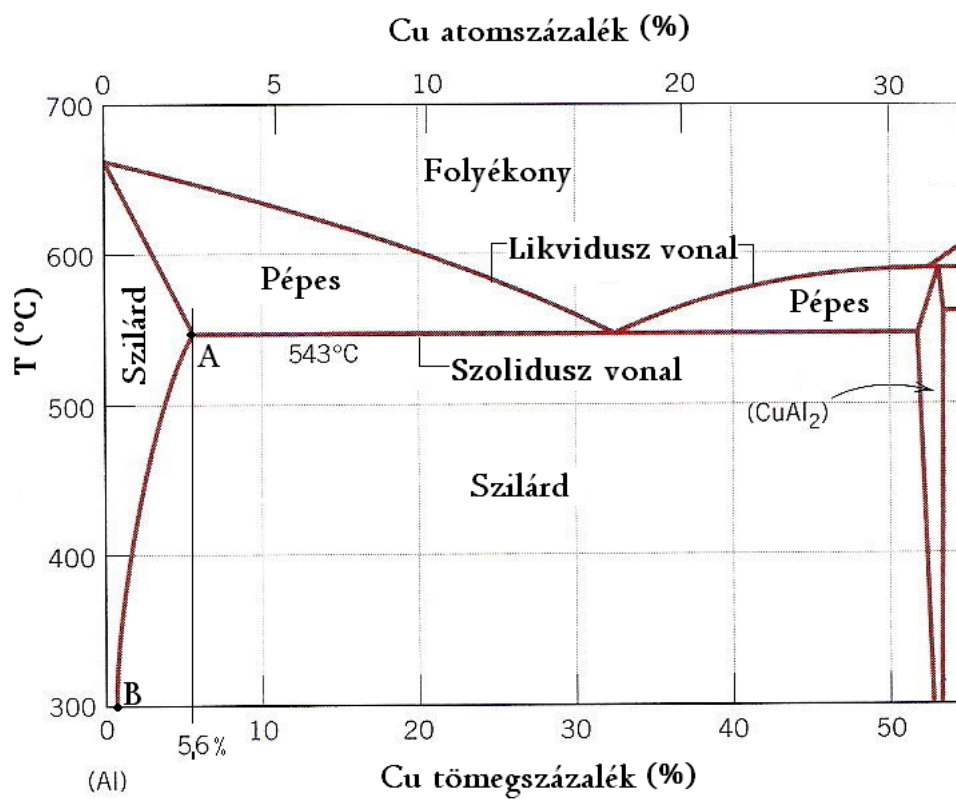
2.21. ábra. Az alumínium-réz (Al-Cu) ötvözetek állapotábrájának egy részlete 54% Cu tartalomig [Csizmazia1], [Jarfas]
