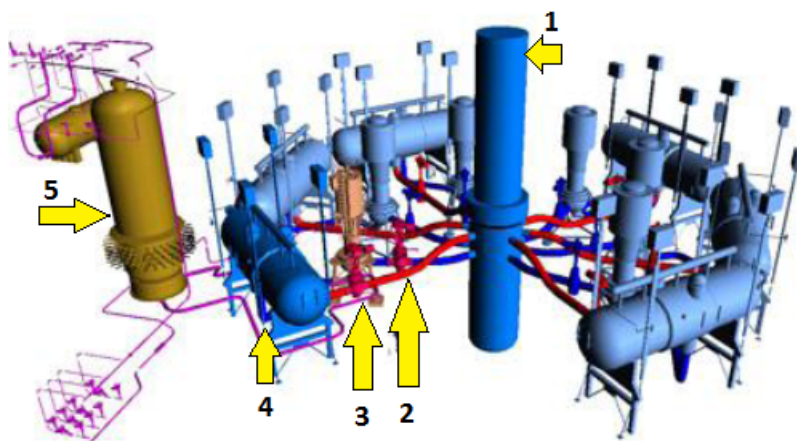
6.4. ábra. A Paksi Atomerőmű primerkörének főberendezései: 1 - reaktor, 2 - főelzáró tolózár, 3 - főkeringtető szivattyú, 4 - gőzfejlesztő, 5 - térfogat kompenzátor [PA Web]
