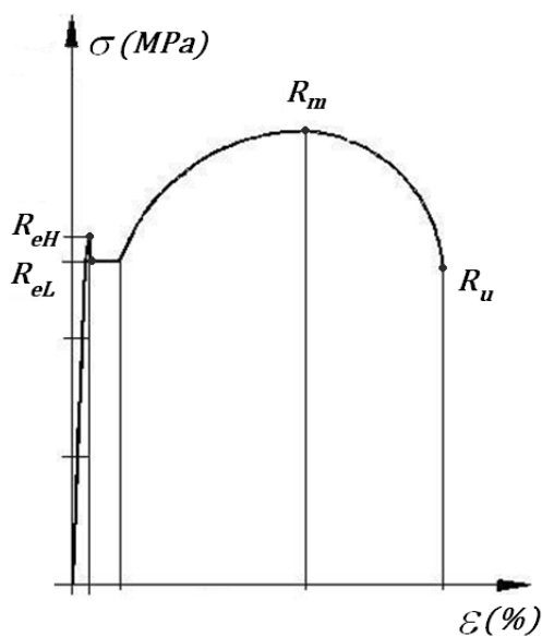
4.7. ábra. A szakítódiagram átszámított, mérnöki feszültség - mérnöki alakváltozás formája [Csizmazia2], [Jarfas]
