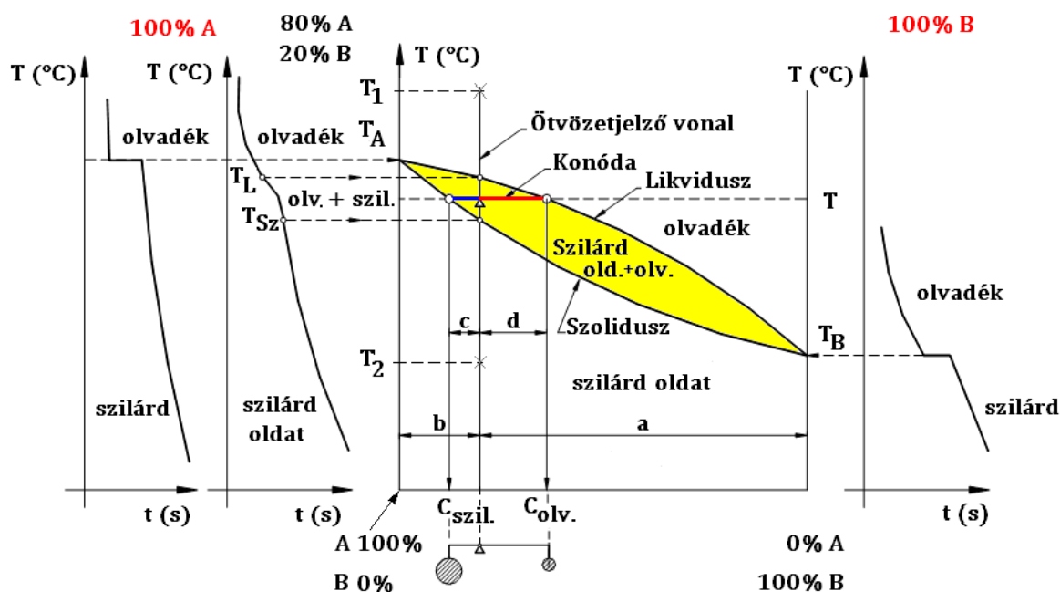
2.16. ábra. Egymást korlátlanul oldó két komponensű ötvözetrendszer állapotábrája és lehülési görbék [Csizmazia1]
