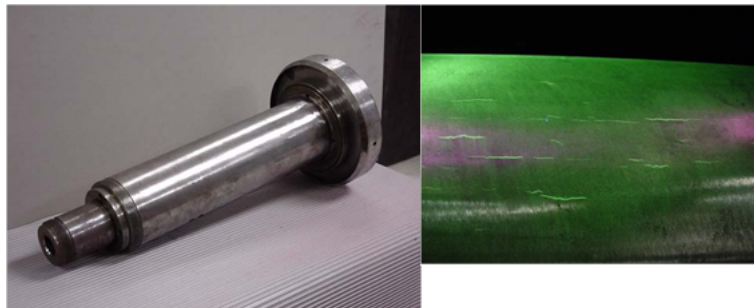
5.13. ábra. Hőkezeléssel keletkezett repedések észlelése fluoreszcens festékkal [NDT web]
