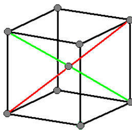
2.2. ábra. Térközepes köbös rács, jele: „TKK” (pl. Cr; W; Mo; Fe; V rácsszerkezete) [Csizmazia1], [Prohaszka]
