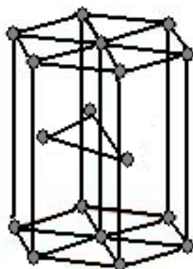
2.4. ábra. Hexagonális rács, jele: „HG” (pl.: Mg; \beta -Ti stb. rácsszerkezete) [Csizmazia1], [Prohaszka]
