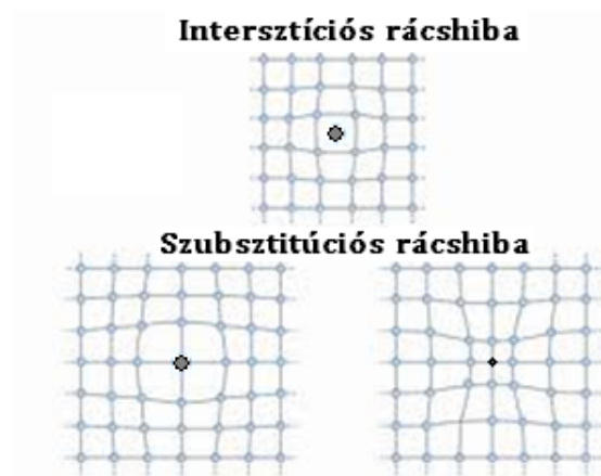
2.6. ábra. A szubsztitúciós és interstíciós szilárd oldat és a bennük jelentkező rácestorzulások [Csizmazia1], [Prohaszka]
