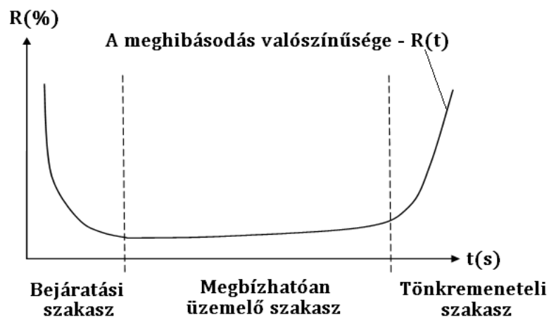
6.2. ábra. Az alkatrészek megbízhatósági függvénye, a kádgorbe [Rajz: Kiss A.]
