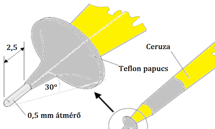
5.45. ábra. A ceruza-teszt (más néven Hsu-Nelson) kalibrálásakor egy 0,5 mm-es grafitceruzát használunk teflon papuccsal [NDT web]
