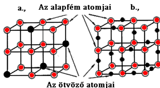
2.11. ábra. Rácsszerkezetek szilárd oldatokban (vegyeskristályokban): (a) szubsztitúciós, (b) interstíciós szilárd oldat [Csizmazia1], [Prohaszka], [Jarfas]
