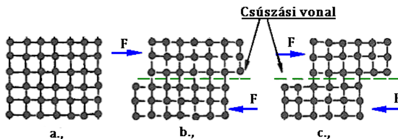
2.12. ábra. Színfém rácsszerkezete (a), a rácselmozdulás vagy csúszás egyszerűsített (az összes kötés nem egyszerre halad!) folyamata képlékeny alakváltozáskor (b és c) [Csizmazia1], [Prohaszka], [Jarfas]
