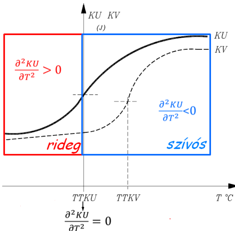
4.15. ábra. A Charpy féle ütvehajlító vizsgálat által meghatározható ütőmunka-hőmérséklet diagram és annak jelentősége, [Csizmazia2]
