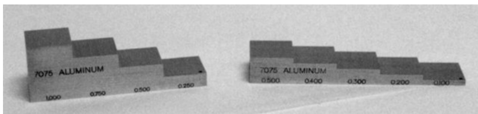
5.25. ábra. A lépcsős etalon [NDT web]
