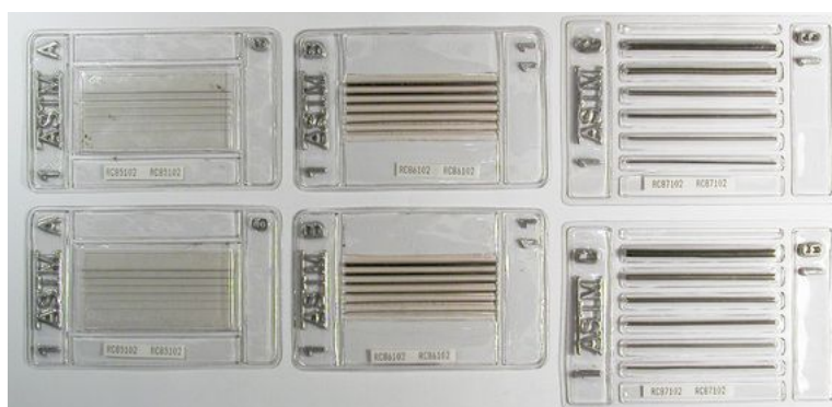
6.28. ábra. Különböző méretű tűsor etalonok. Alkalmazásuk a vizsgált anyag minőségétől, vastagságától függ, segítségükkel megállapíthatjuk az alkalmazott paraméterekkel kimutatható hiba méretét [Ke-Tech Kft web]
