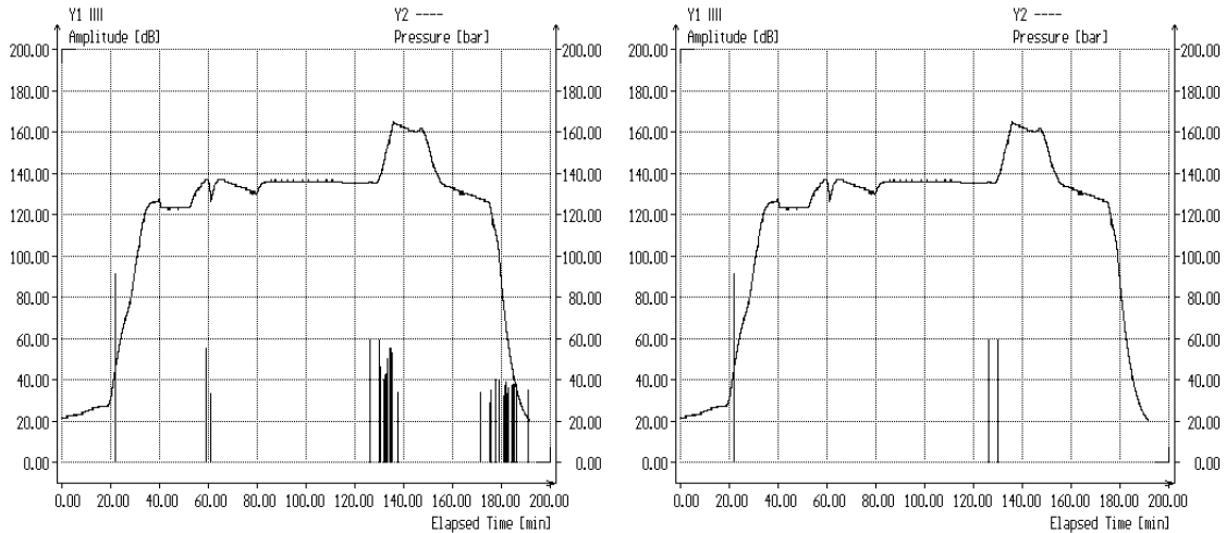
6.37. ábra. Az akusztikus emissziós események a reaktortartály nyomáspróbája során. Balra: 21 dB-nél nagyobb események, jobbra: 56 dB-nél nagyobb események [KFKI AEKI]
