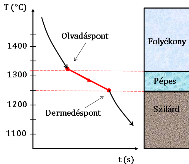
2.10. ábra. Az ötvözet lehűlési görbéje [Csizmazia1], [Prohaszka], [Jarfas]
