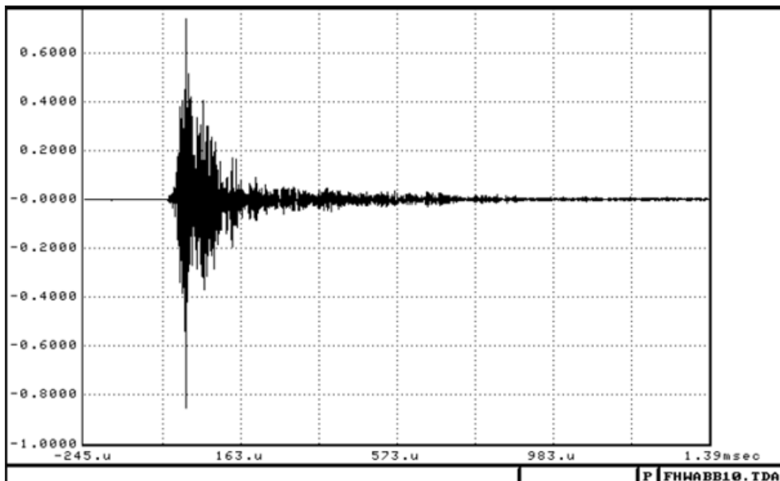
5.33. ábra. Egy tipikus akusztikus emissziós "börst" [NDT web]: a függőleges tengelyen az amplitúdó, a vízszintesen az idő
