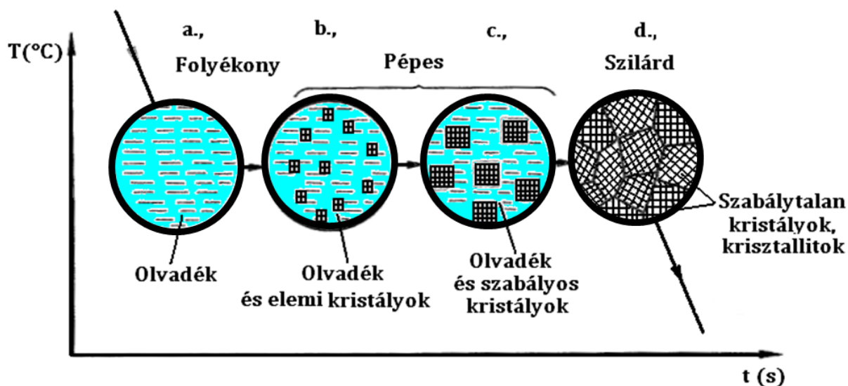
2.8. ábra. A fémek kristályosodásának folyamata [Csizmazia1], [Prohaszka], [Jarfas]
