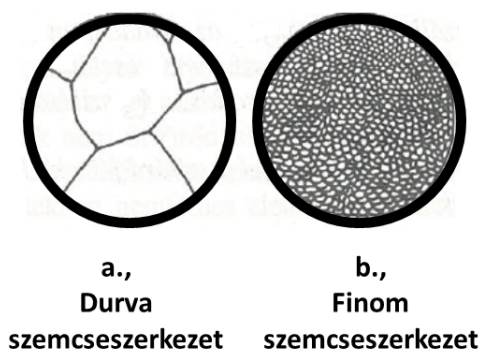
2.9. ábra. A durva (a) és finom (b) szemcseszerkezetű színfém mikroszkópi képe [Csizmazia1], [Prohaszka]), [Jarfas]
