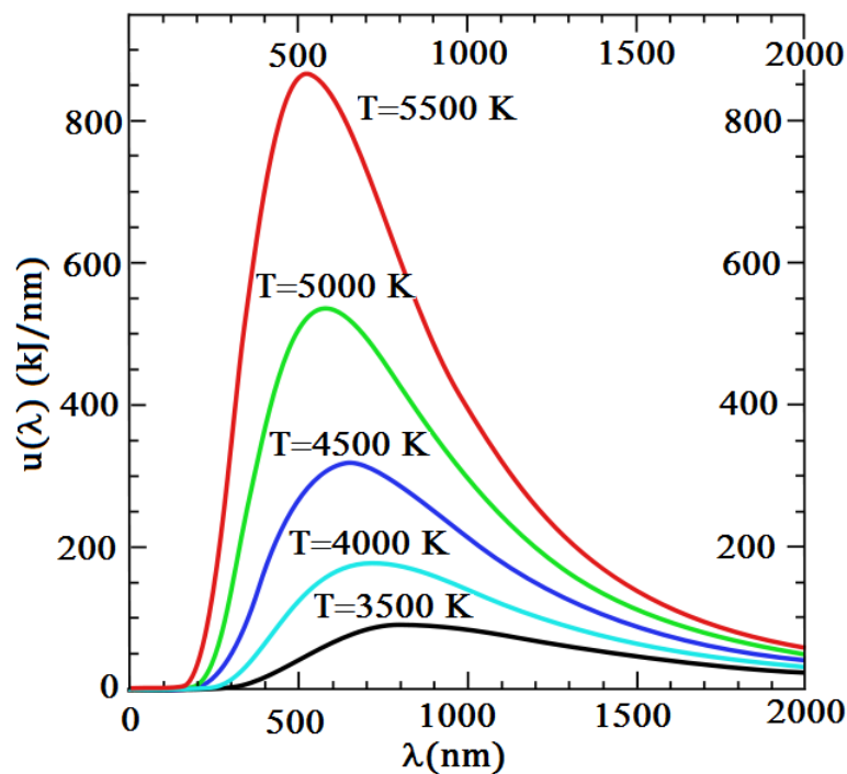
5.46. ábra. A fekete test Planck féle sugárzási törvénye grafikusán ábrázolva [Rajz: Kiss A.]
