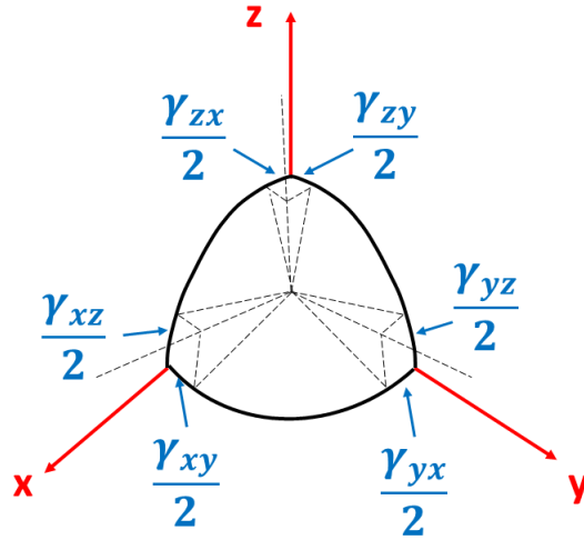
3.2. ábra. Az alakváltozási állapot szemléltetése [Rajz: Kiss A.]
