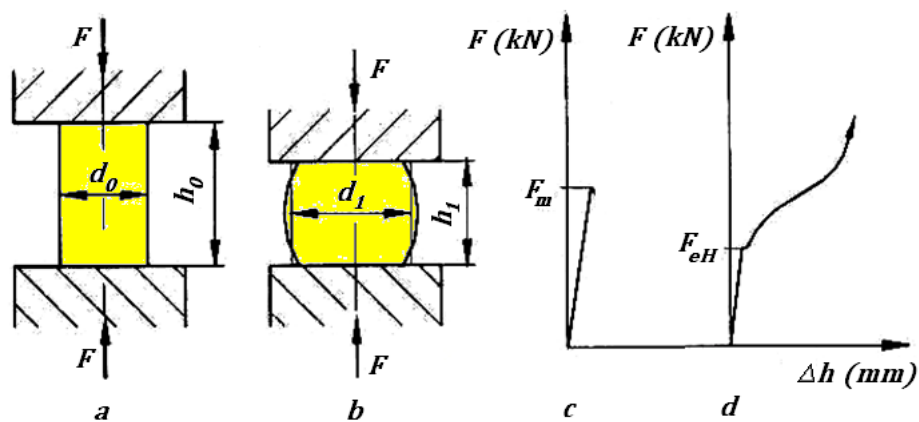
4.9. ábra. Az anyagok viselkedése nyomó igénybevétel során: a, terheletlen-, b, terheelt mintadarab és méretei, c, rideg anyag-, d, szívós-képlékeny anyag nyomódiagramja, [Csizmazia2]
