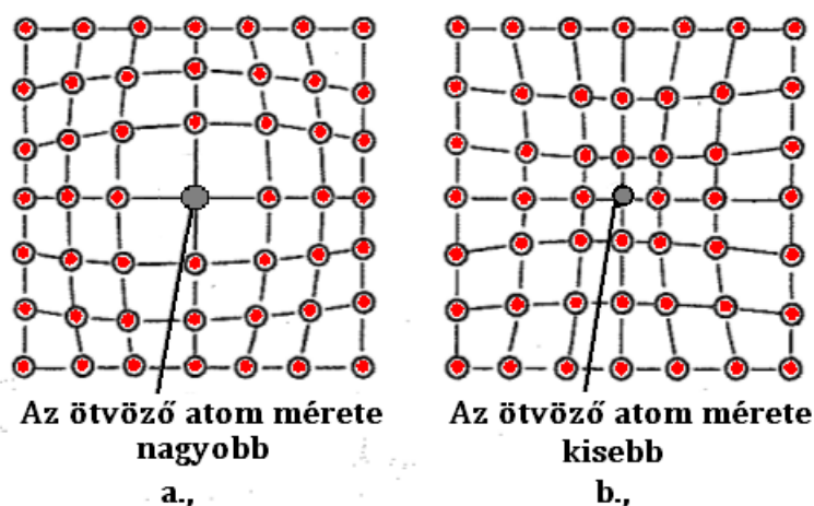
2.14. ábra. Jellemző ráctorzulások szilárd oldatok kristályrácsába: a, esetben az ötvöző atom mérete nagyobb, mint az alapfémé. b, esetben az ötvöző atom mérete kisebb, mint az alapfémé [Csizmazia1], [Prohaszka], [Jarfas]
