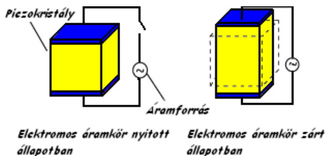
5.20. ábra. Az elektrostrikciónak elve [NDT web]
