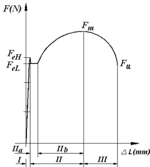
4.5. ábra. A lágyacél szakítódíagramja [Csizmazia2], [Jarfas]
