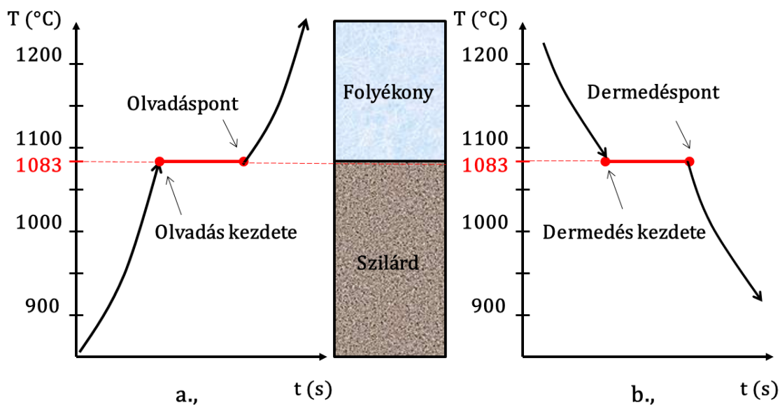
2.7. ábra. A színfémek (jelen esetben réz) felmelegítési (a) és lehűlési (b) görbéje [Csizmazia1], [Prohaszka]), [Jarfas]
