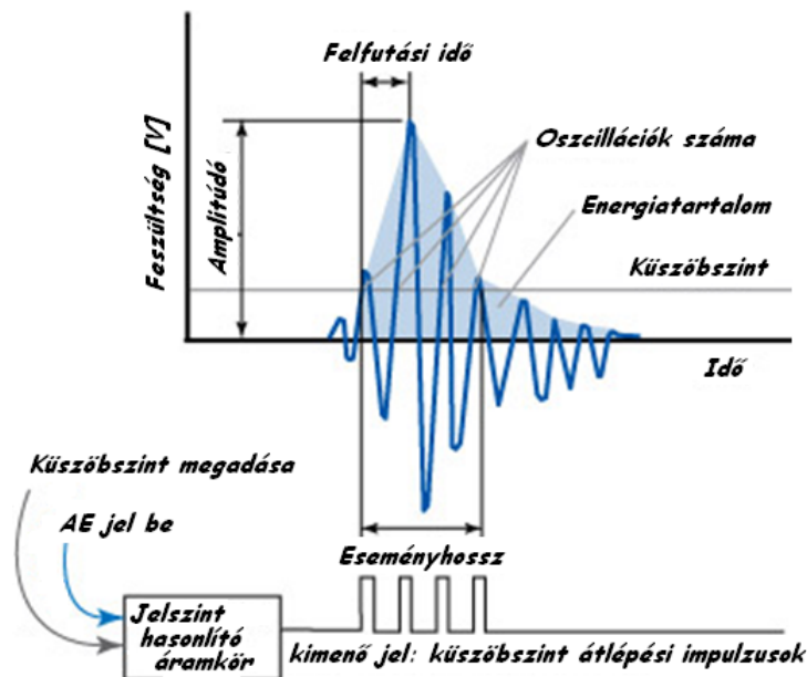
5.34. ábra. Az akusztikus emissziós "börzst" jellemző mennyiségei [NDT web]
