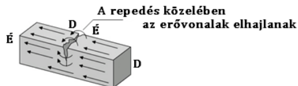
5.5. ábra. A mágneses repedésvizsgálat elve [NDT web]
