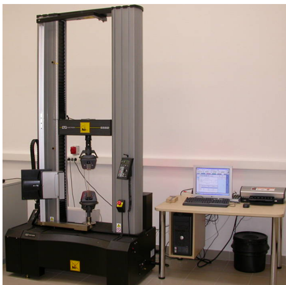
4.2. ábra. Egy korszerű szakítógép [Csizmazia2]
