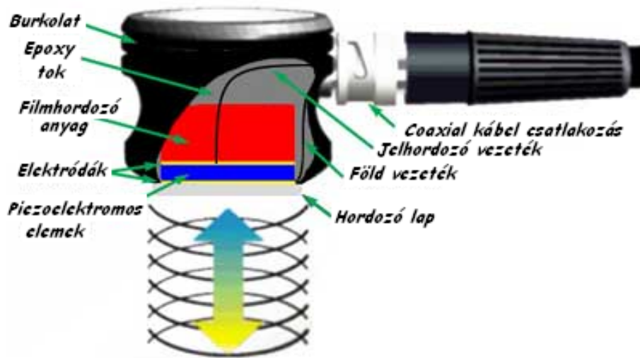
5.21. ábra. Egy piezoelektromos vizsgálófej keresztmetszete [NDT web]
