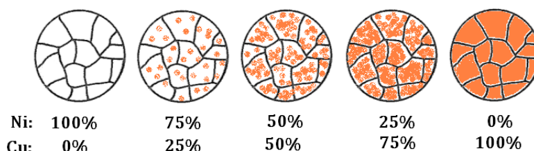
2.19. ábra. A réz-nikkel (Cu-Ni) ötvözetek szövetszerkezeti képe különböző százalékos összetételnél [Csizmazia1], [Jarfas]
