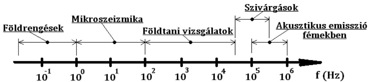
5.28. ábra. Akusztikus frekvenciaspektrum [Pellionisz] [Rajz: Kiss A.]
