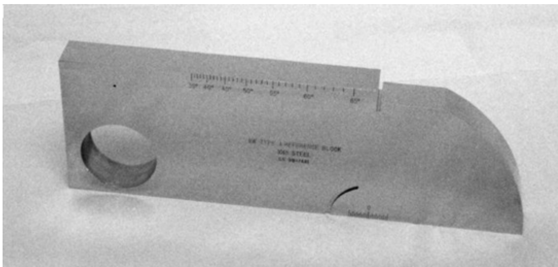
5.23. ábra. Az ET1 etalon [NDT web]
