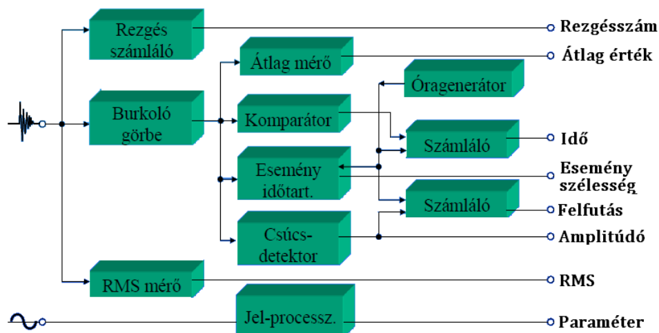
5.38. ábra. Egy egycsatornás készülék általánosított blokkdiagramja [Rajz: Gemes Gy.]
