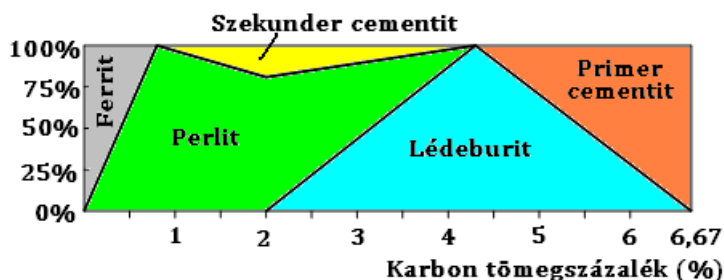
2.25. ábra. A vas - vas-karbid ( Fe - Fe_3C ) ötvözetek szövetdiagramja 20^\circ\text{C} -on [Csizmazia1], [Jarfas]
